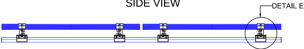
Klip-lok bracket
